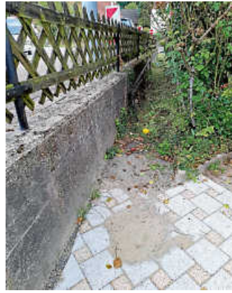
Die Stützwand hat sich bereits geneigt. Foto: Stadt Gaggenau
